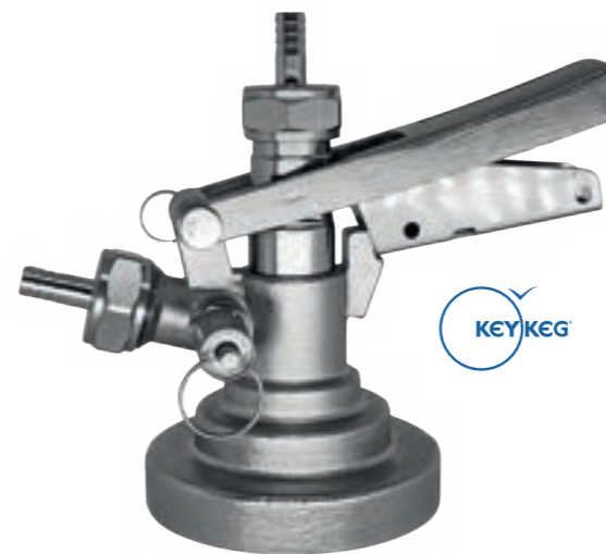
HBS1011-24 Extrator tipo F (tipo KeyKeg®) Completa
