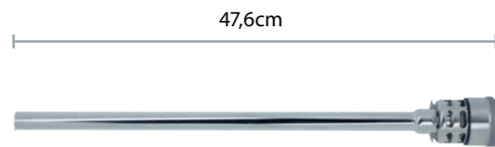
HBS0334-50 Sifão Tipo S Inox p/barril 50L, sem trava
