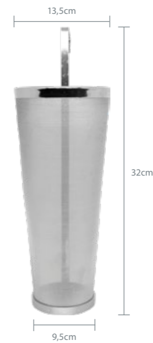
HBS0030-03 Filtro cônico com alça 300 micra Ø superior 13,5cm Ø inferior 9,5cm Altura: 32cm
